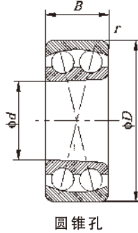
圆锥孔
