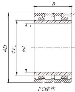
FC结构
