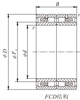
FCD结构
